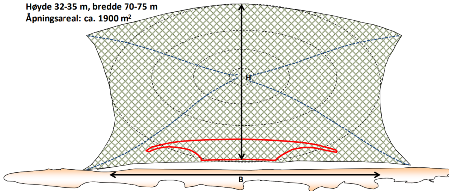
Figur 17 – Dimensjon av en bunntål og en pelagisk trål sett forfra (Fiskeridirektoratet, 2013).
