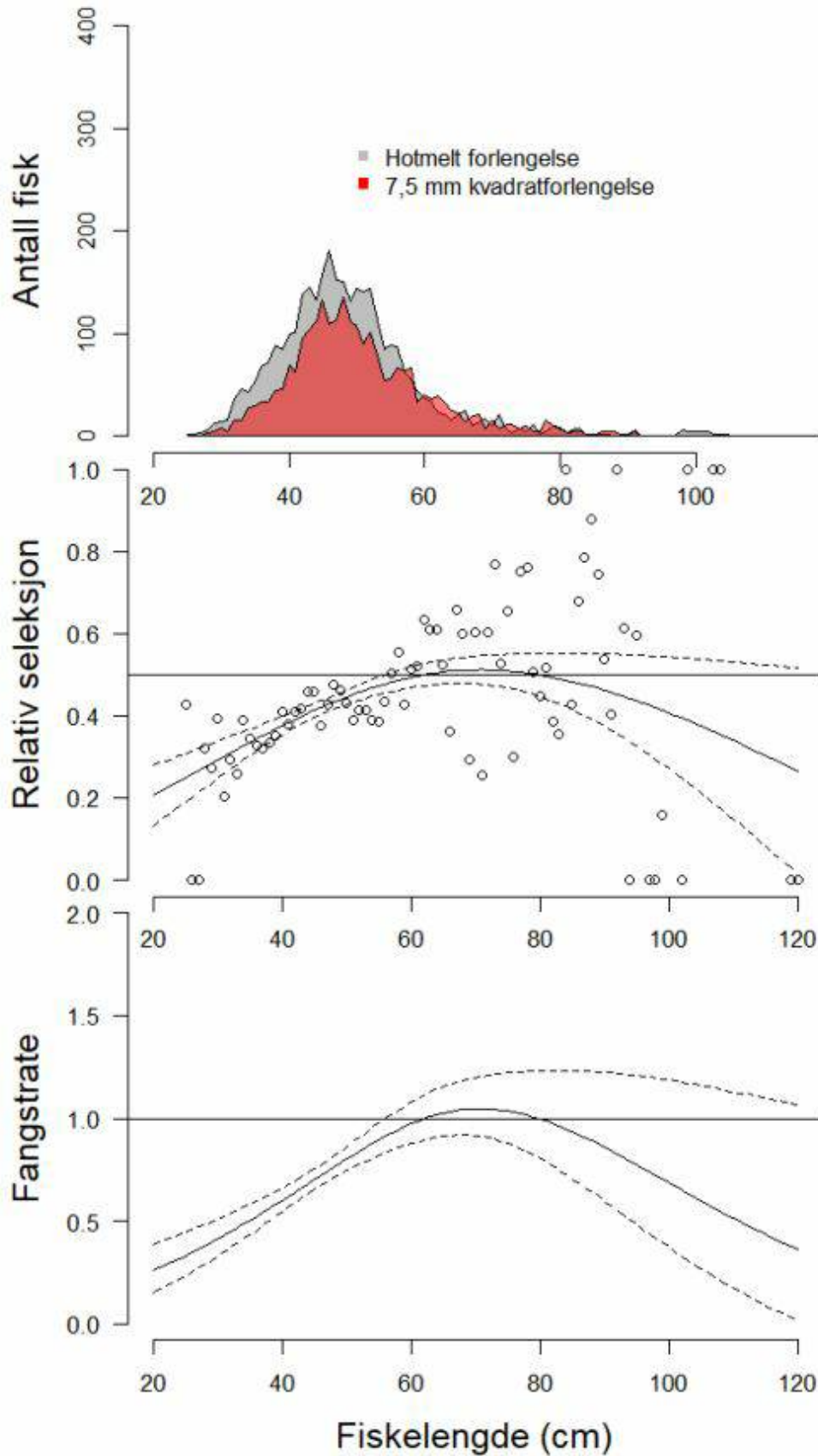
Figur 11 . Størrelsesfordelinger for torsk i hver forsøksserie (topp) med 7 parvise hal. Relativ fangst i snurrevadsekk med 7,5 mm tråd i kvadratmaskeforlengelse, sammenlignet med sekk med diamantmaskeforlengelse (midt). Figuren nederst viser relativ fangstrate (fangsttap av fisk < ca 60 cm) ved å bruke kvadratmaskeforlengelse.
