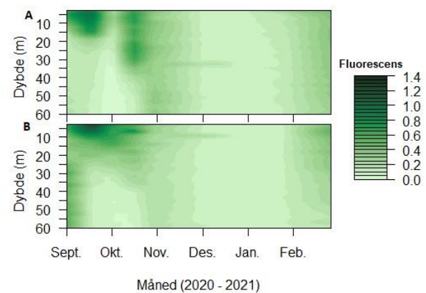
Figur 6: Interpolerte fluorescensprofiler ( \mu\text{g l}^{-1} ) fra september 2020 til mars 2021 ved lokalitetene A og B fra 0 til 60 meters dybde.
