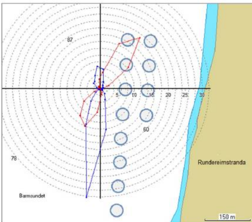
Figur 2.1.3 Kart med strømrose (% relativ flux) på målepunktet: målt ved 5m og 15m vandndyp
