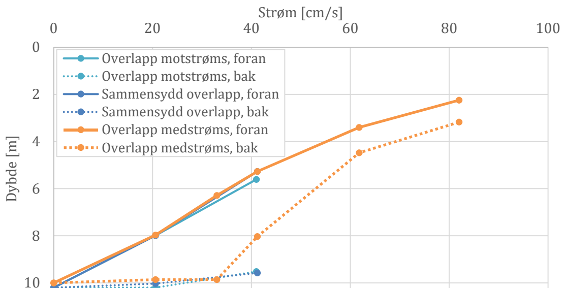
Figur 18. Skjørtedyptet foran og bak (vertikal akse med vannflaten ved 0) med hensyn på strøm hastigheten (horisontal akse) for konfigurasjonene spissnot med 10 m tett skjørt med overlapp medstrøms, motstrøms og sammensydd i skjøten.
