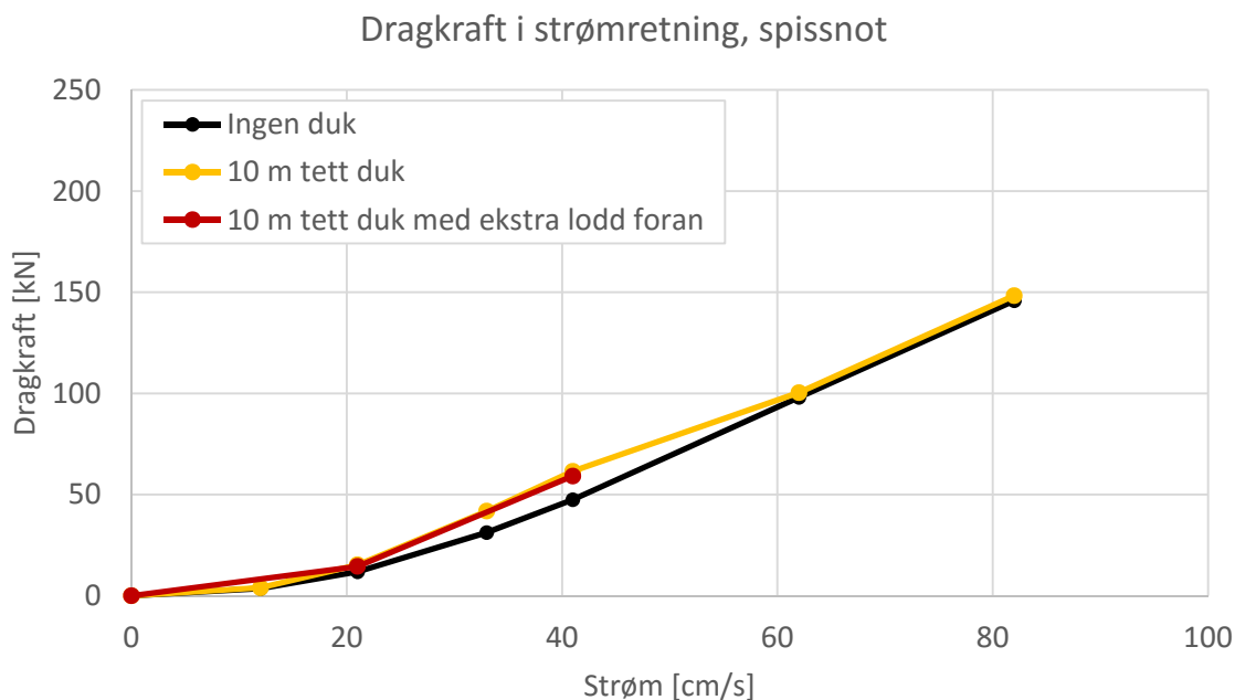
Figur 14. Dragkrefter parallelt med strømmen (vertikal akse) med hensyn på strømhastighet (horisontal akse) for konfigurasjonene spissnot uten skjørt, med 10m tett skjørt og 10 m tett skjørt påmontert et lodd på 100 kg i front oppstrøms.
