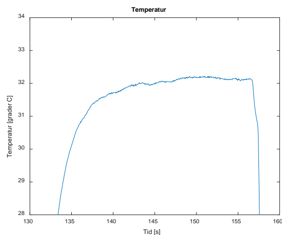
Figur 10, utsnitt temperaturprofil i termisk avluser
