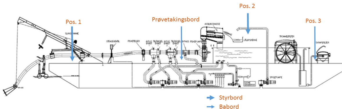
Figur 4 – Prinsippskisse for Hydrolicer LG9332 Hydro versjon 3 med seks parallelle (like) linjer. Laks i avkast pumper inn (venstre side). Fisken passerer fisketeller, to seriekoblede enheter for lusfjerning (basert på avsugning og trykksetting av vann), en Aqua-Life Biostream BP120 fiskepumpe per linje som så løfter fisken opp til en silkeasse der fisk og prosessvann separeres. Fisken går til merd i en delvis vannfylt renne og prosessvannet går til trommelfiltre som separerer ut fast stoff som lus og skjell. Figuren viser også hvor det ble tatt ut fisk til evaluering. Posisjon 1 – Fisk før avlusning ble håvet fra merd til vannfylte kar for senere prøvetaking og evaluering stress, velferd og lusetall. Posisjon 2 – Fisk etter avlusing ble behandlet på samme måte. Posisjon 3 – Fisk tatt ut ved utløp til merd (kun ved innledende forsøk) der den avlusede fisken ble håvet direkte fra rennen. Avlivet fisk ble båret fra Posisjon 1-3 til et arbeidsbord for analysearbeid plassert under tak midt på lekteren. Kilde: MNH
