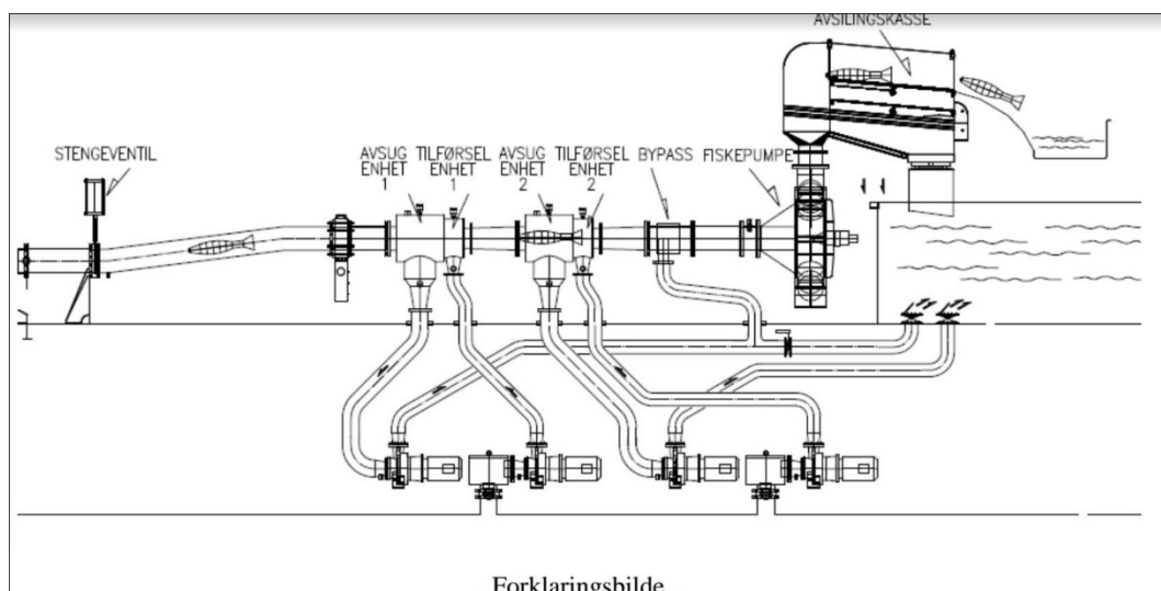
Figur 5 – Forstørret figur som viser de to seriekoblede enhetene for lusfjerning, fiskepumpen og silkassen som separerer fisk og prosessvann. Hver enhet for avlusing har egen krets for henholdsvis avsugning og tilførsel av trykksatt. Hydrolicer versjon 3 har seks slike system i parallell for å øke kapasiteten av fisk til avlusing. Fiskens bevegelsesretning er fra venstre mot høyre. Kilde: MNH.
