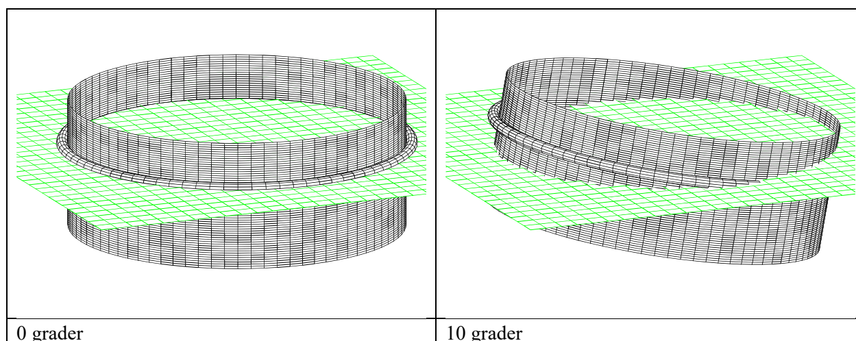
Figure 8: Reduksjon av opprettende moment på grunn av neddykking av flytekrage.
