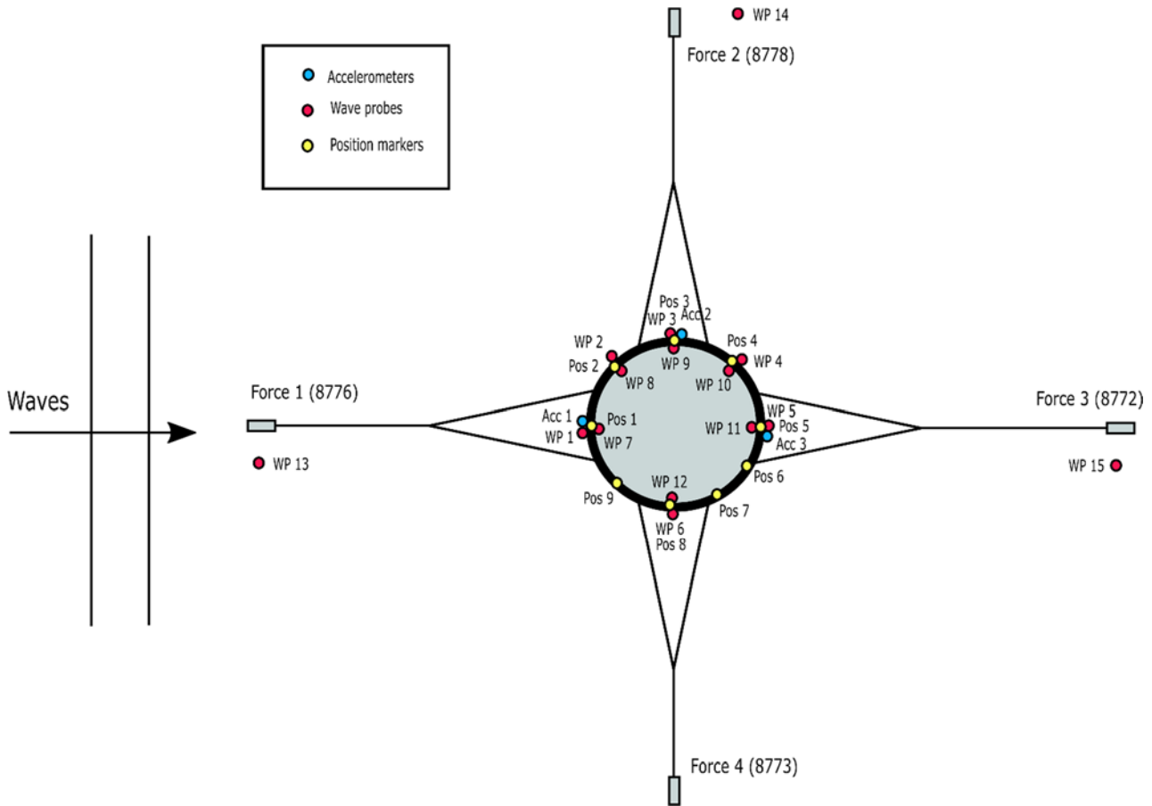
Figure 3: Instrumentering av merdmodell. Plassering av akselerometere, posisjonsmarkører (oqus), bølgemålere og lastseller.
