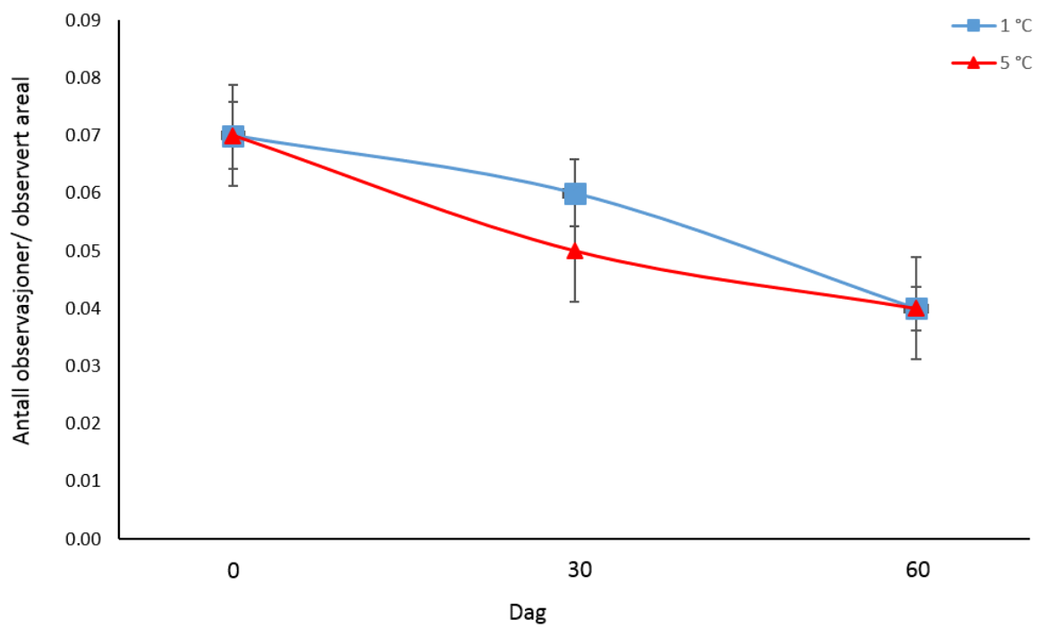
Figur 5 Endring i vakuolisering i hepatopankreas fra snøkrabber holdt ved 1 °C og 5 °C ved dag 0, 30 og 60. Hvert punkt (n=5) viser gjennomsnittet ±SEM
