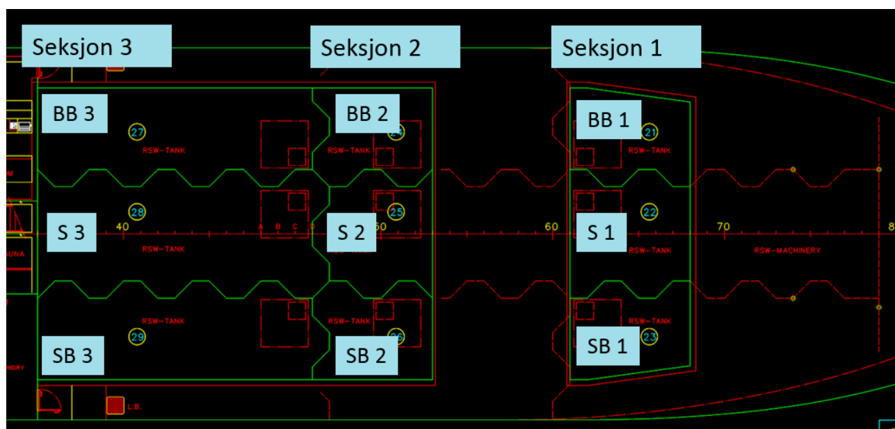
Figur 1. Plassering av RSW-tankene i "Selvåg Senior". BB 3 = babord seksjon 3, BB 2 = babord seksjon 2, BB 1 = babord seksjon 1, S 3 = senter seksjon 3, S 2 = senter seksjon 2 og S 1 = senter seksjon 1.
