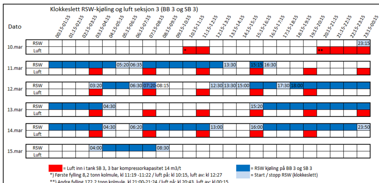
Figur 17. Oversikt over luftkjøring og RSW-kjølesykluser i seksjon 3 fra 10. til 15. mars
