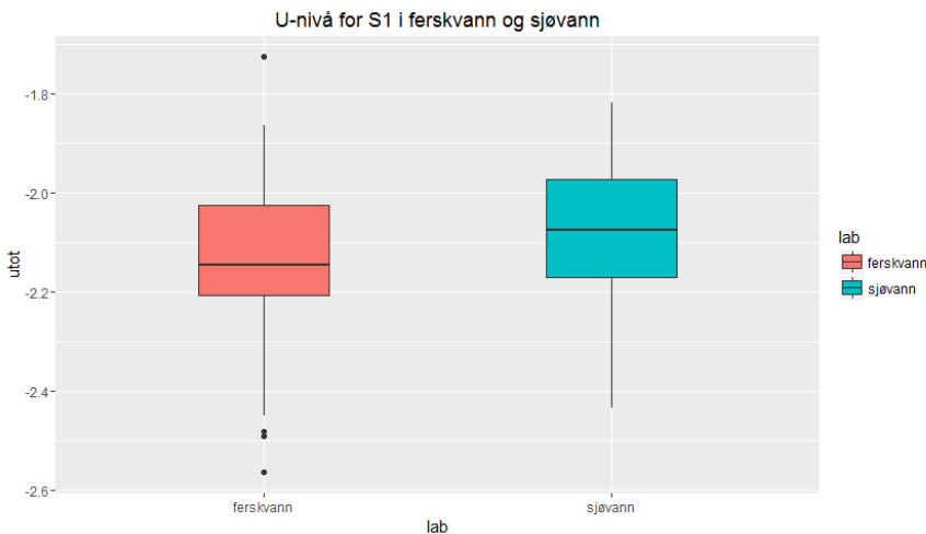
Figur 7. Boksplokk for U-nivå log(mg/kg) for S1 i ferskvann og etter 2 måneder i sjø
