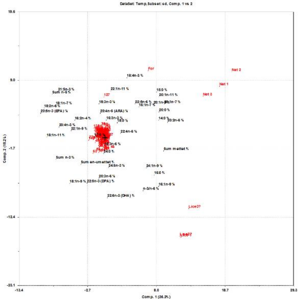
Fig. 10. Principal komponent analyse (PCA) av fettsyreprofil i plasma hos rognkjeks, sammenlignet med fettsyreprofil i lus, nettgroe og fôr.
