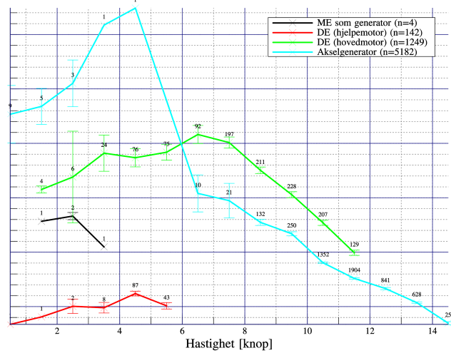
Figur 7: Gjennomsnittlig normalisert forbruk som funksjon av hastighet for ulike propulsjonsmoder, for driftssituasjoner med typisk thrustnivå og elektrisk konsum mellom 350 og 400 kW. Figuren viser ett plott for hvert av fartøyene. Hver linje korresponderer til en driftsmodus. For eksempel er rød linje dielelektrisk drift med hjelpemotor som energikilde. Tallene angir hvor mange minutter måling som inngår i hvert punkt og hver linje. Lengden på de vertikale strekene angir konfidensintervall, som kan sees på som forholdet mellom variasjon i målingene og antall målinger. Se forklaring til propulsjonsmoder i teksten.
