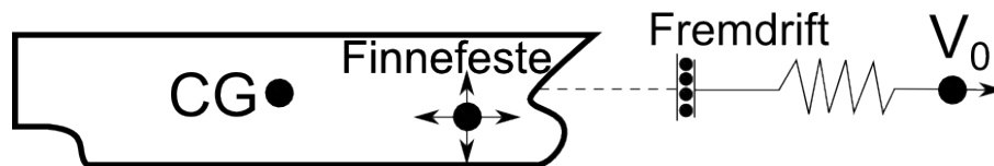
Figur 5: Simuleringsoppsett med fremdriftskraft generert av en fjær som beveger seg med fast fart V_0 som gjennomsnittlig fart
