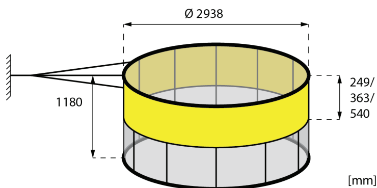
Fig. 3.2.2. Nøkeldimensjoner for modellmerden. Skjørtet ble prøvd ut med tre forskjellige dybder, henholdsvis 249, 363 og 540 mm.
