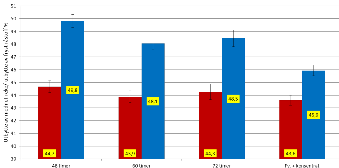
Figur 11. Røde søyler viser gjennomsnittlige pilleutbytter for modnet reke ved ulike tid i kald modningslake, og blå søyler viser beregnede pilleutbytter av fryst reke (+/- standardavvik).
