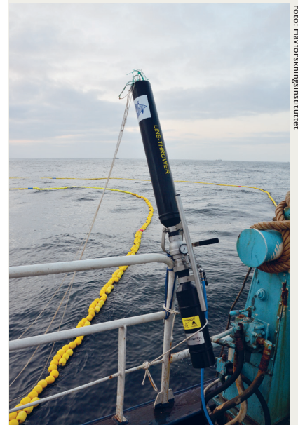
Figur 2. Luftkanon for utskyting av prøvetakingstrål.
