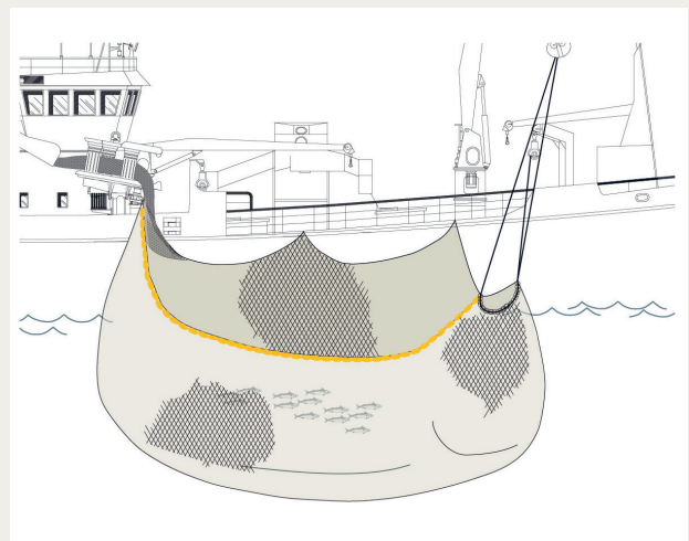
Figur 4. Not rigget med rundstropp gjennom "geila".
