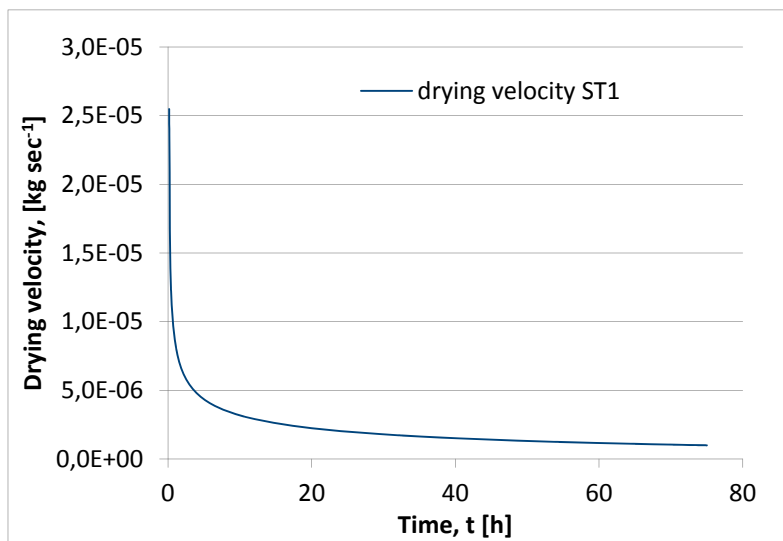
Figur 4: Gjenomsnittlig tørkehastighet av en klippfisk som funksjon av tørketid
