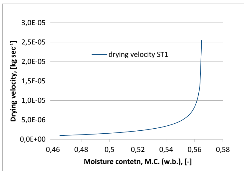
Figur 5: Gjenomsnittlig tørkehastighet for en klippfisk som funksjon av fuktinnhold
