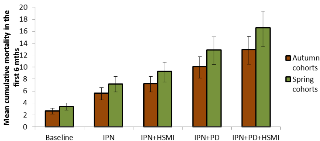
Figur 26 Gjennomsnittlig kumulativ dødelighet for de første 6 månedene i sjø for vår og høstsmolt under ulike scenarier. I alle scenariene var vekt ved sjøsetting satt til medianen (107g), og temperatur ved sjøsetting var 9.3°C (median). Variasjonslinjene viser hhv 10 % og 90 % temperatur ved sjøsetting. År=2012.
