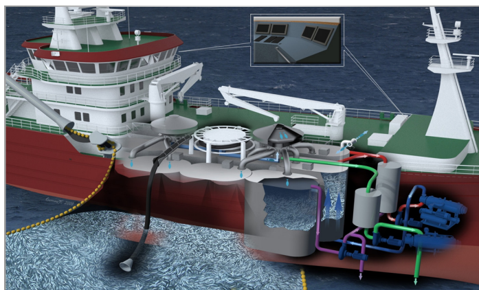
Figur 1: Konsepttegning for undertrykklasting (Ref. MMC)
