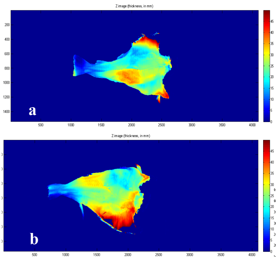
Figur 11 – Kalibrert 3D-bilde i dimensjon 'mm'. Bildet er fargekodet for å vise lokale høydeforskjeller på klippfisken. Økende rødhet betyr større høydeforskjeller, mens de blå fargetonene betyr lavere høydeforskjeller (transportbåndet har nivå lik 0 mm). (a) En 'superiorfisk', og (b) en 'sortidofisk'.
