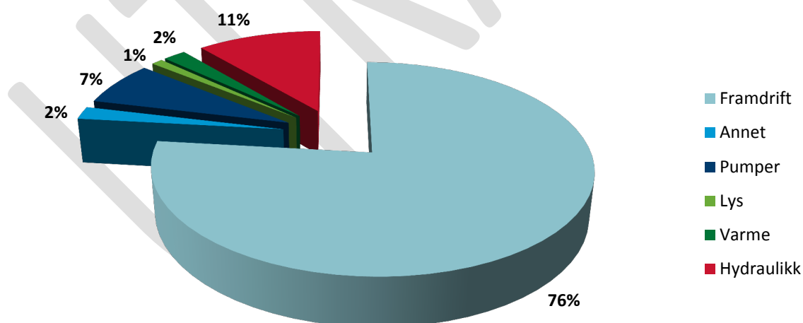
Figur 3.7 Energiforbruk per energibruker for kystfiskefartøy som drifter med snurrevad (Jenssen, 2011)
