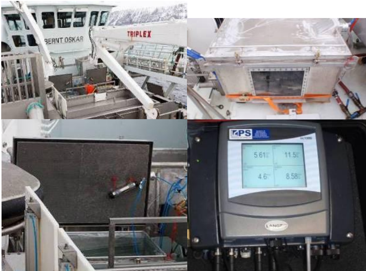
Figur 2.2.1. Oppe venstre: plassering av kar om bord på ”Bernt Oskar”; Oppe høyre: lukket kar med fisk, justering av vanngjennomstrømming; Nede venstre: plassering av oksygenmåler i lokk før avsilingsrist. Nede høyre: overvåking av oksygen og temperatur fra loggeenhet.
