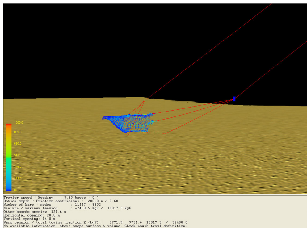
Figur 1 Datasimulering av ny bunntrål fra Vonin P/F som blir holdt oppe av pelagiske tråldører. © Vonin P/F.
