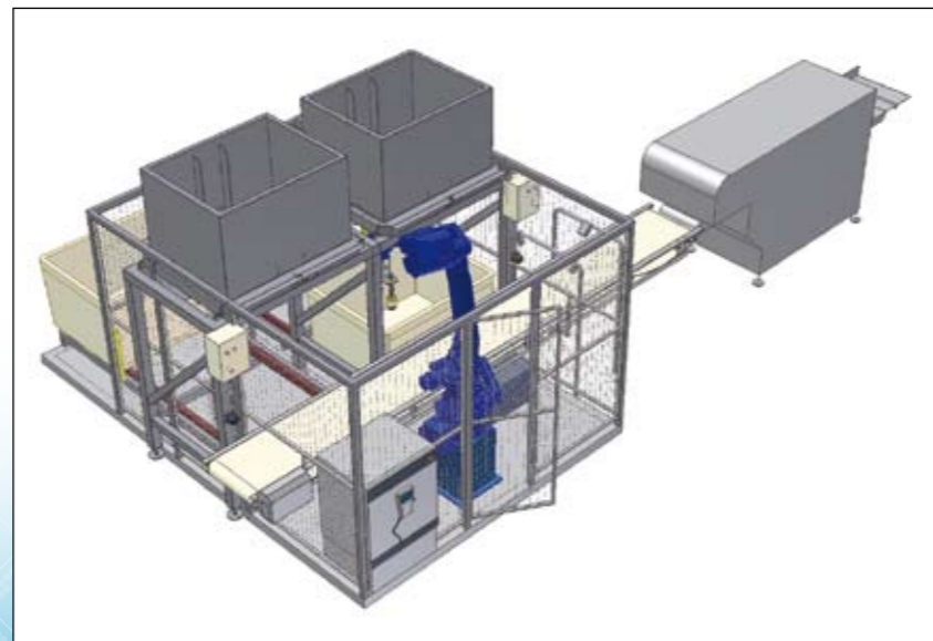
3D modell av robotcelle for salting av fisk i kar
