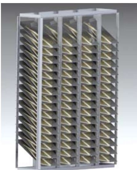
Fig. 3: Bufferlager for klippfisk (Magasin)
