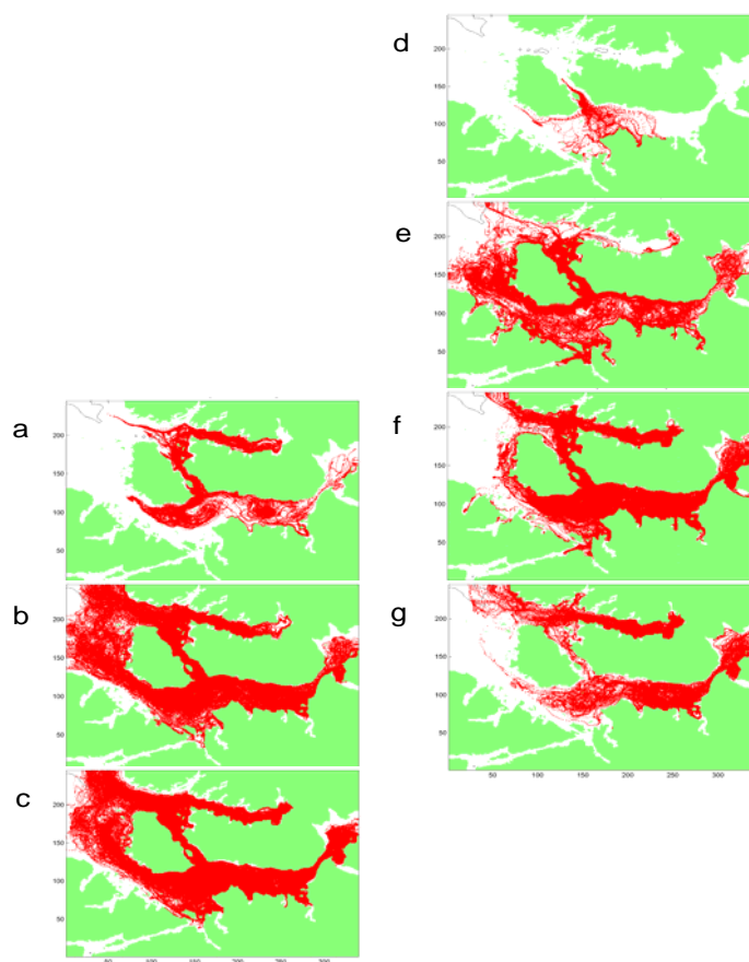
Figur 8. Partikkelbesøk fra partikler sluppet fra lokalitet 5 i Hadselsundet, i a ) mai 1999, b ) juni 1999, c ) juli 1999, d ) mars 2000, e ) april 2000, f ) mai 2000 og g ) juni 2000 (Brørs og Slagstad 2004).
