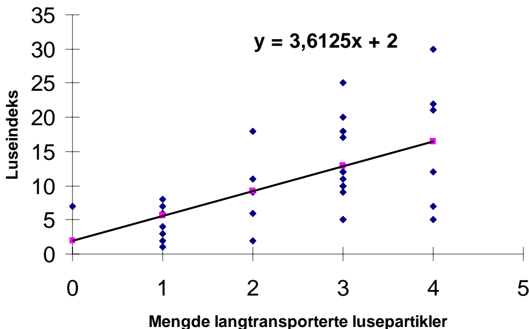
Figur 14. Figuren viser forholdet mellom mengden langtransporterte lusepartikler (hentet ut fra simuleringsmodellen) og luseindeks på oppdrettsfisk ( r^2=0.32 ; p<0.001 )(Figuren modifisert fra Koren 2005).
