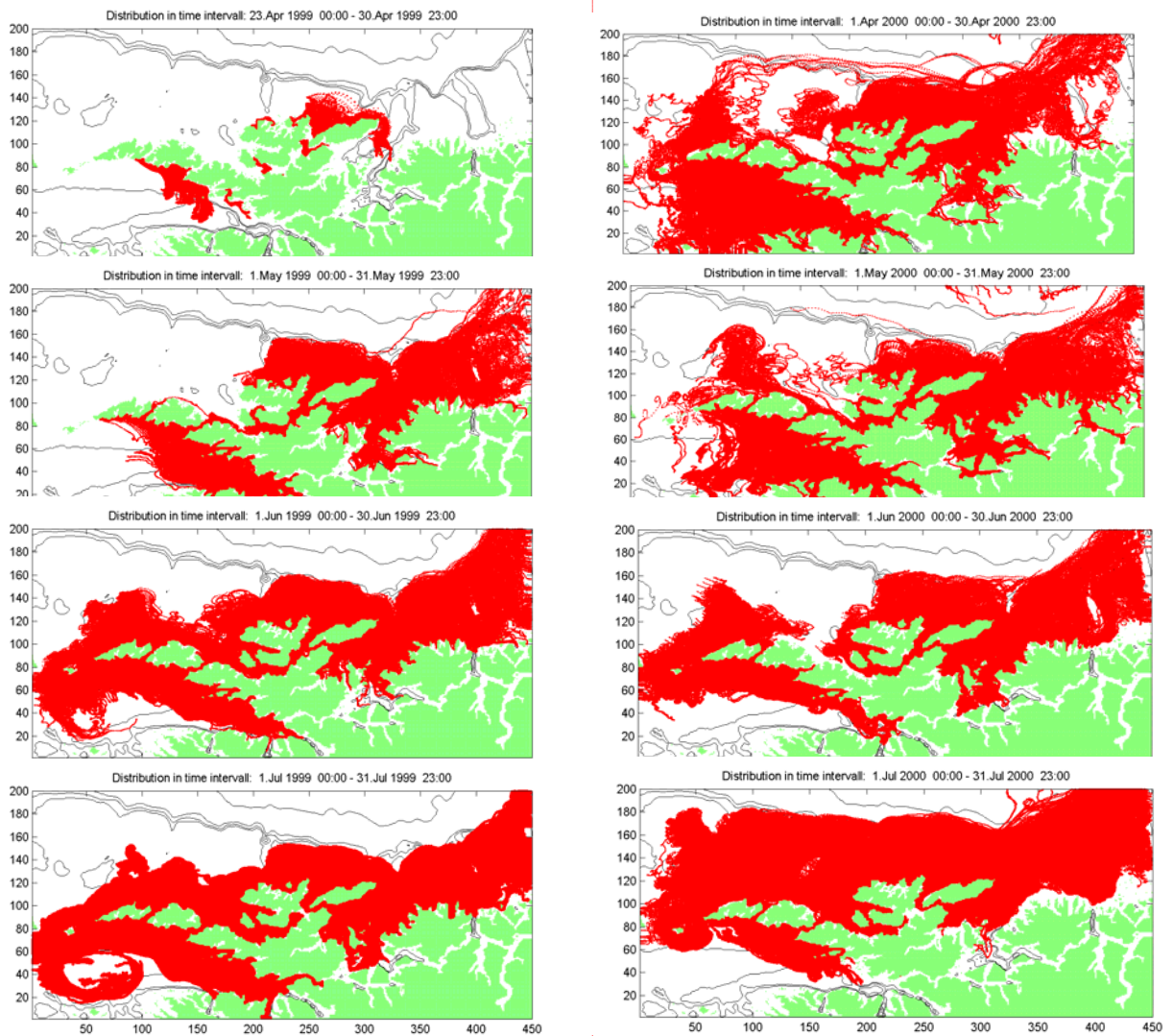
Figur 3. Røde felt viser områder som har hatt besøk av en partikkel sluppet fra en av lokalitetene 1-8. Venstre panel viser partikkelbesøk i månedene april – juli 1999, og høyre panel viser partikkelbesøk i samme periode i 2000 (Brørs og Slagstad 2004).
