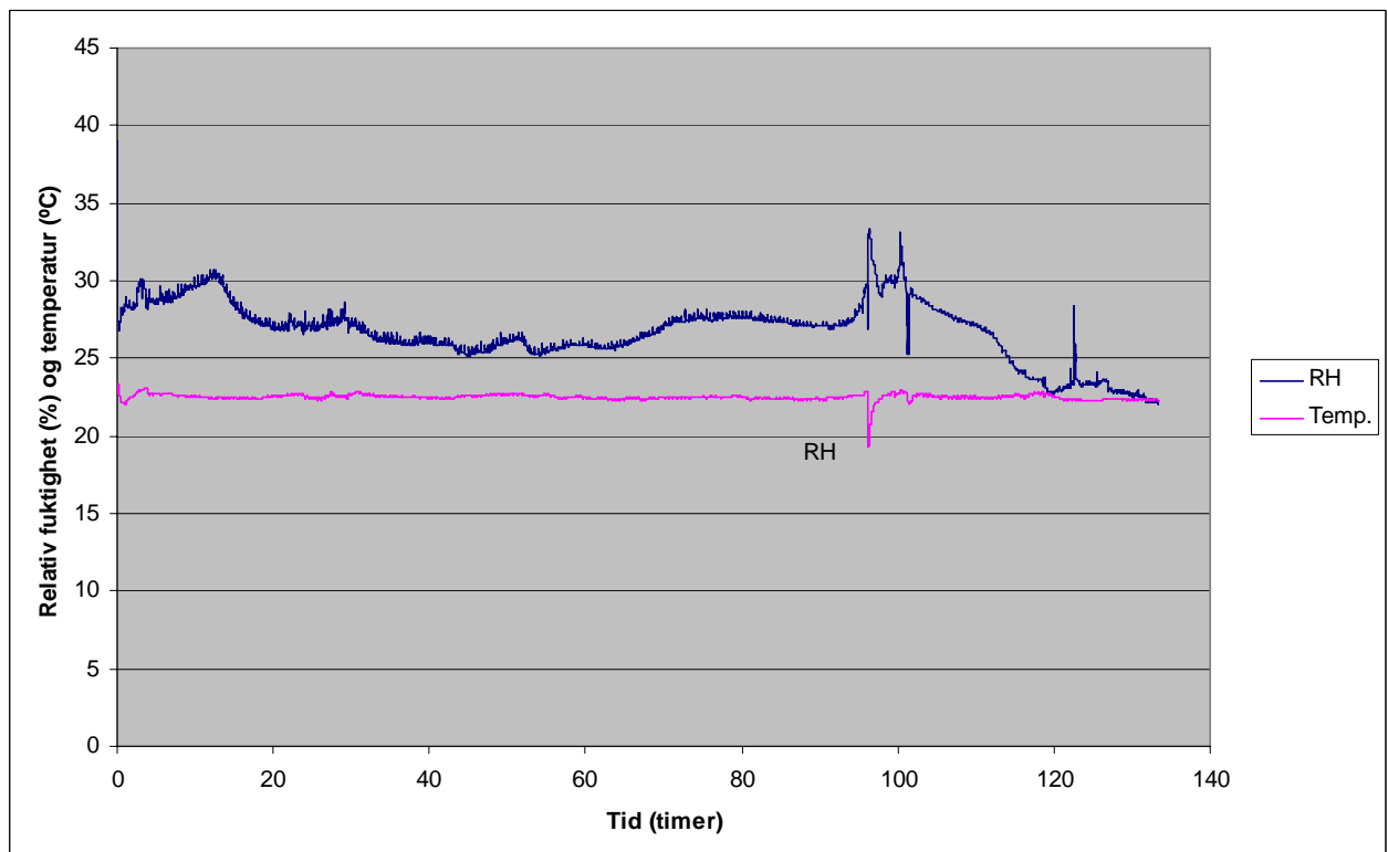
Figur 3 Eksempelkurver fra logging av relativ fuktighet og temperatur undertørking av saltfisk av torsk på lager ved romtemperatur.
