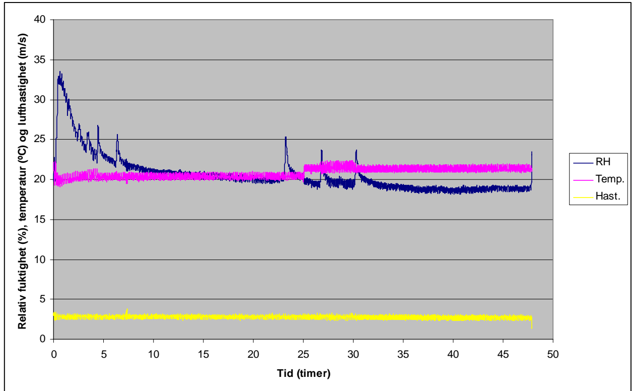
Figur 2 Eksempelkurver fra logging av relativ fuktighet, temperatur og lufthastighet under tørking av saltfisk av torsk i brettørke.
