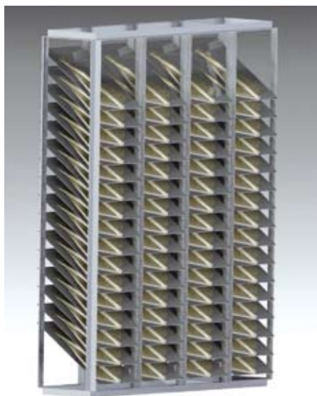
Fig. 3: Bufferlager for klippfisk (Magasin)
