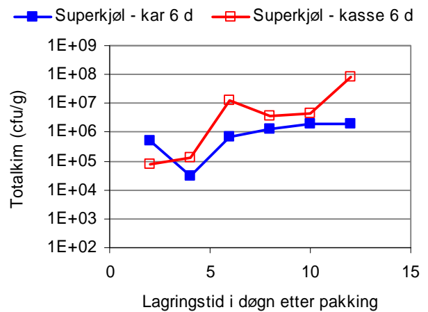
Figur 18. Totalt kimtall i vanlig iskjølte og superkjølte torskeloins produsert av 3 døgn eller 6 døgn gammelt råstoff, kjølt i kar eller iset i kasser før filetering og pakking.
