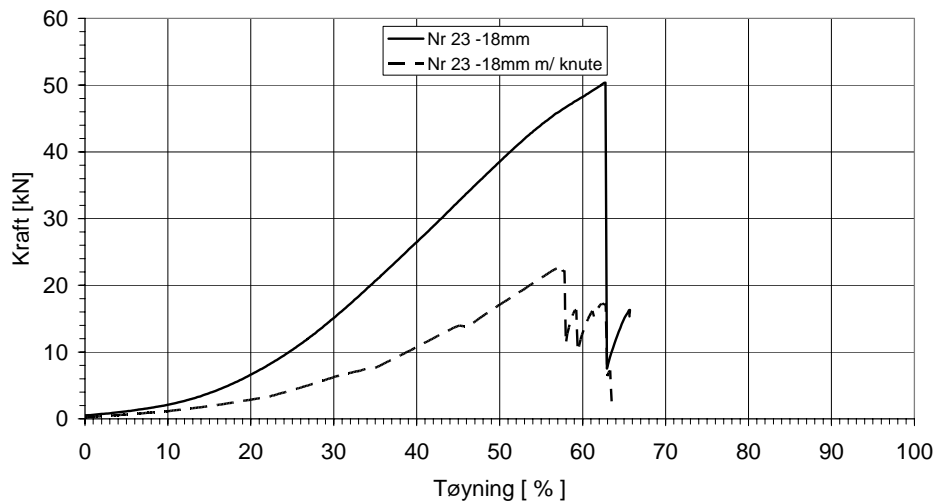
Fig. 6 Endring i bruddlast pga. knute på tauet
